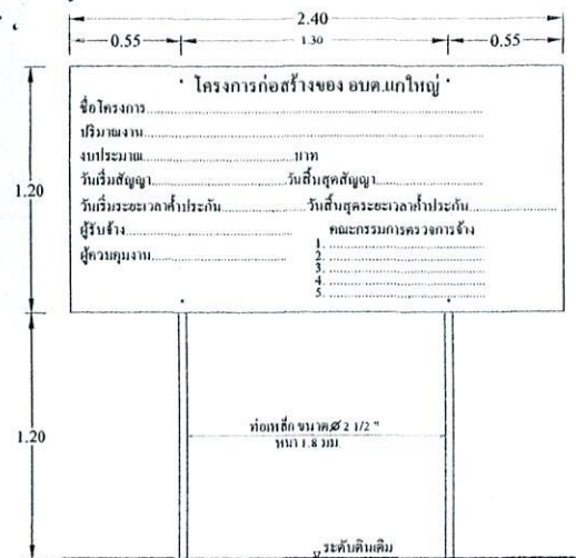
รูปด้านหน้า 1 : 25
